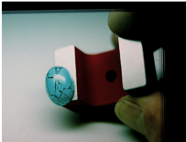
Abb2.: Magnetismus beim Türkis
